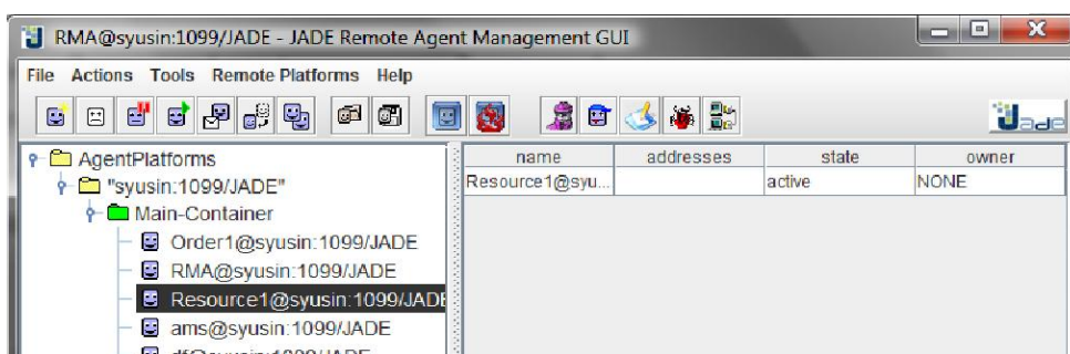
Рис. 5 Инициализация агента
