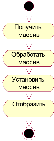
Рис. 39. Диаграмма активности
