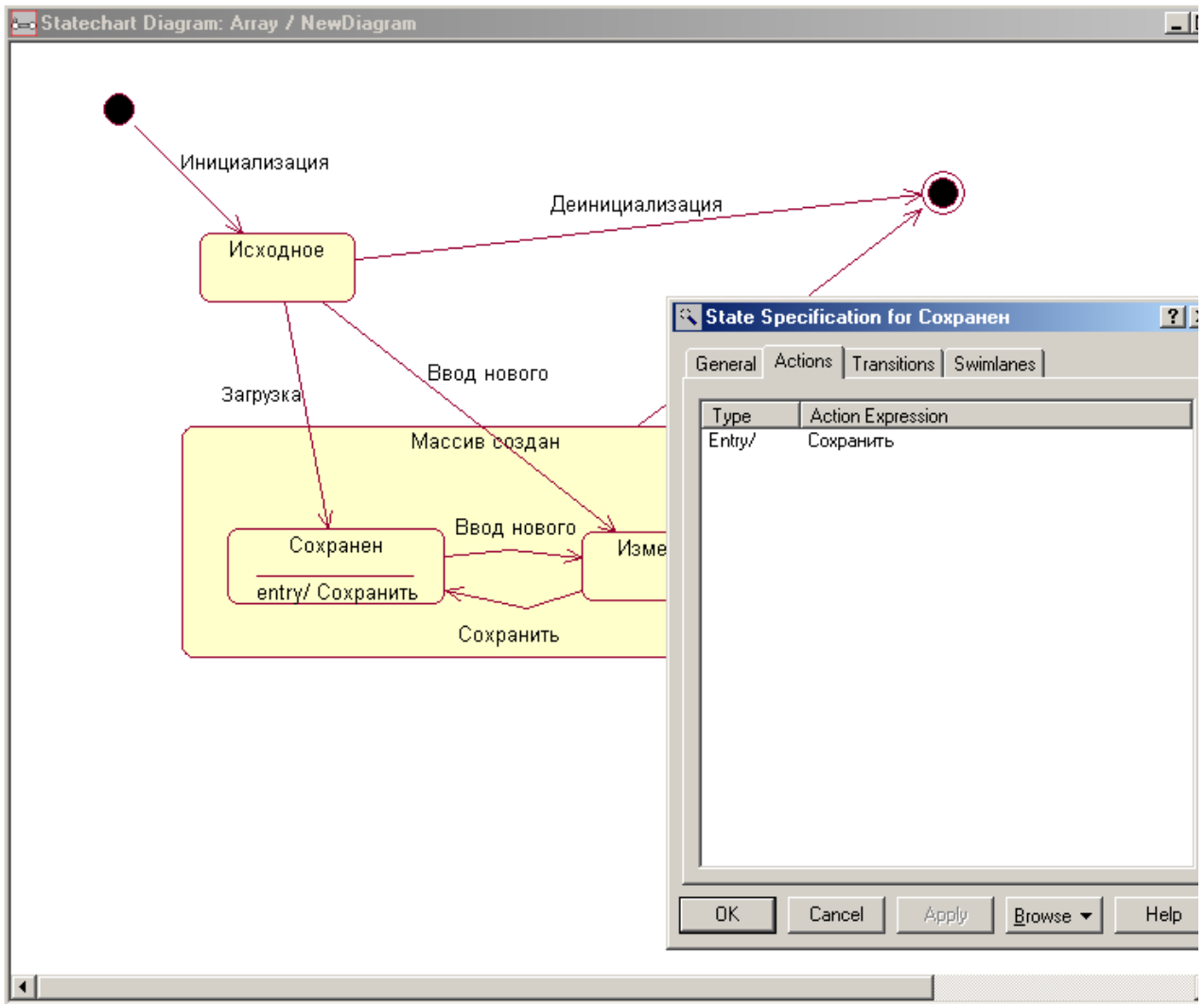
Рис. 37. Состояние с указанными действиями
