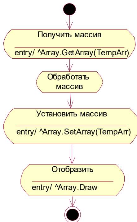
Рис. 40. Диаграмма активности
